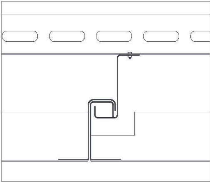
DETAY/DETAIL 1 ÖLÇEK/SCALE 1/2
